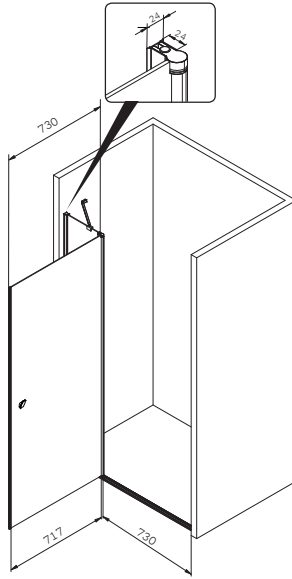
Zweiwegeöffnung two way opening реверсивное открытие
